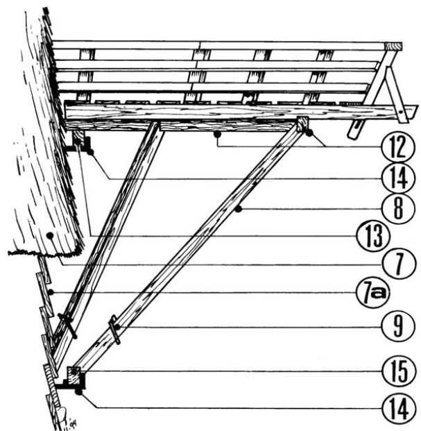
Stelling met sluitingen
