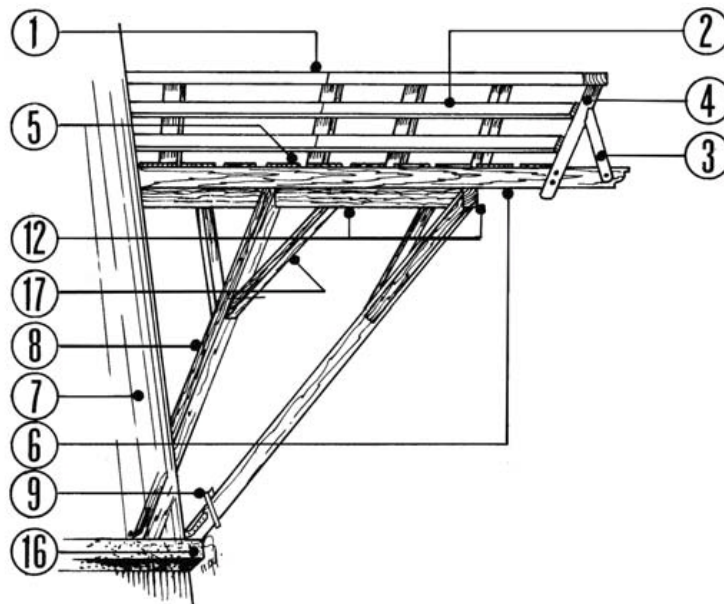
Groninger variant op de stelling
