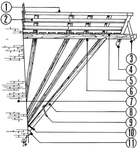
Stelling met onder iedere ligger een schoor
